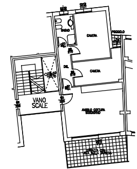
TIPOLOGIA UNITA' Pianta - Tipo F Scala 1:100
