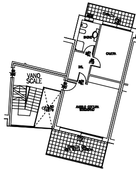
TIPOLOGIA UNITA' Pianta - Tipo B Scala 1:100
