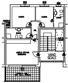
TIPOLOGIA UNITA' Pianta - Tipo D Scala 1:100
