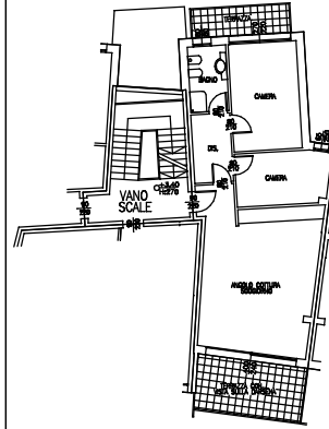
TIPOLOGIA UNITA' Pianta - Tipo E Scala 1:100
