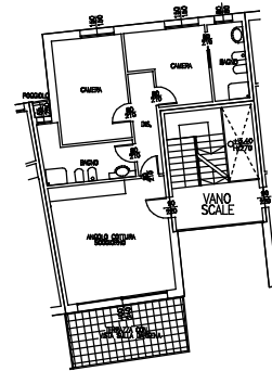
TIPOLOGIA UNITA' Pianta - Tipo G Scala 1:100
