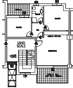
TIPOLOGIA UNITA' Pianta - Tipo C Scala 1:100
